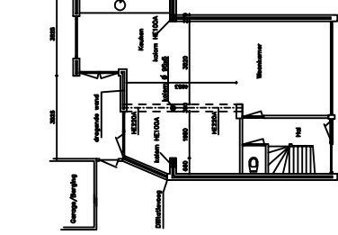
BEGANE GROND GEWIJZIGD.
