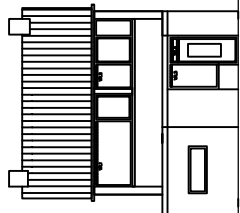
Achtergevel GEWIJZIGDE SITUATIE
