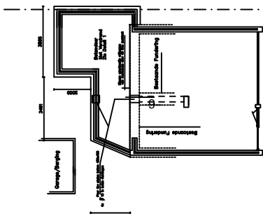
FUNDERING GEWIJZIGD.
