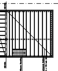
BALKLAAG ZOLDERVLOER GEWIJZIGD.
